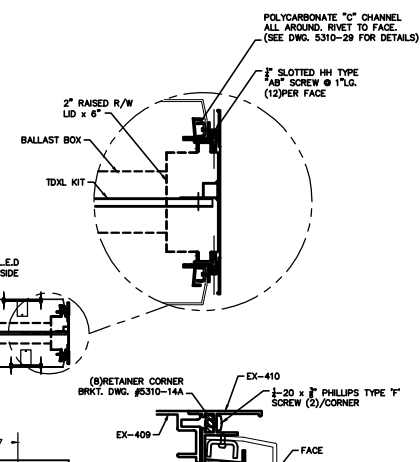
SECTION D-D
