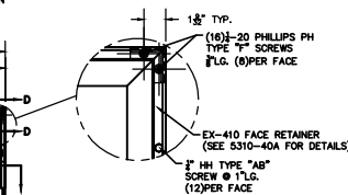
SECTION D-D
