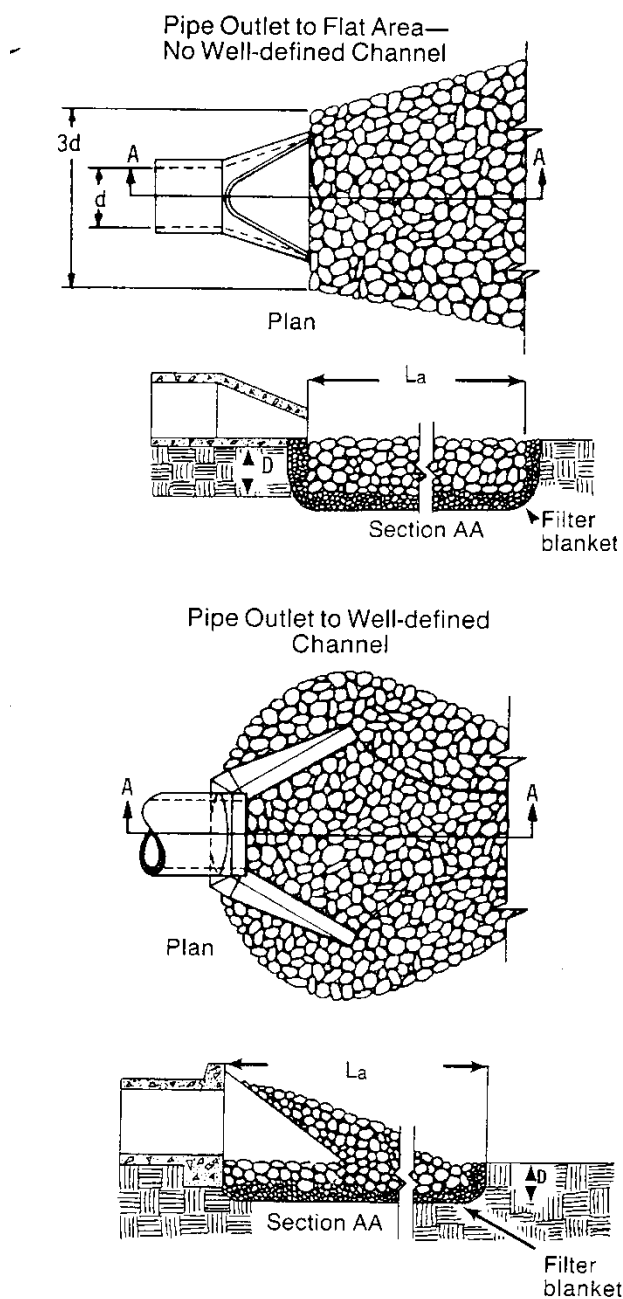
Figure 4.4 Riprap Apron
